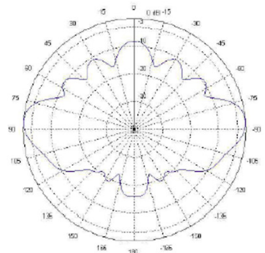
E-Plane
